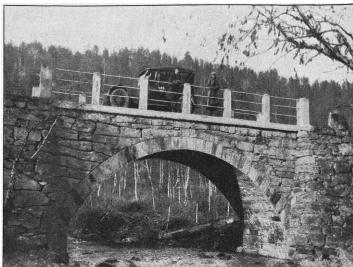
Bro over Anselven (Fagerlidal).
